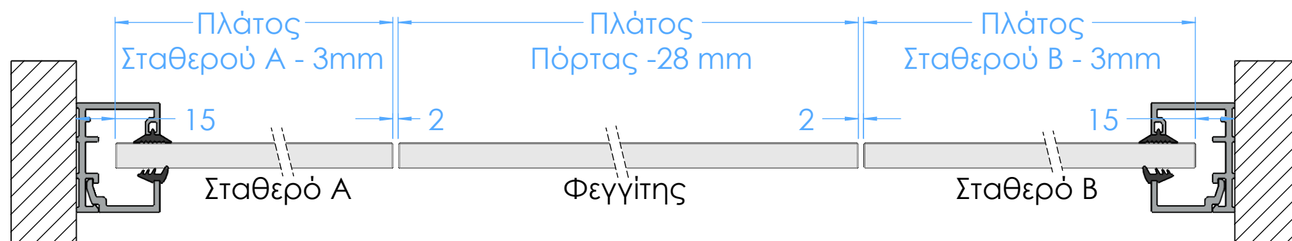
ΤΟΜΗ K-K
