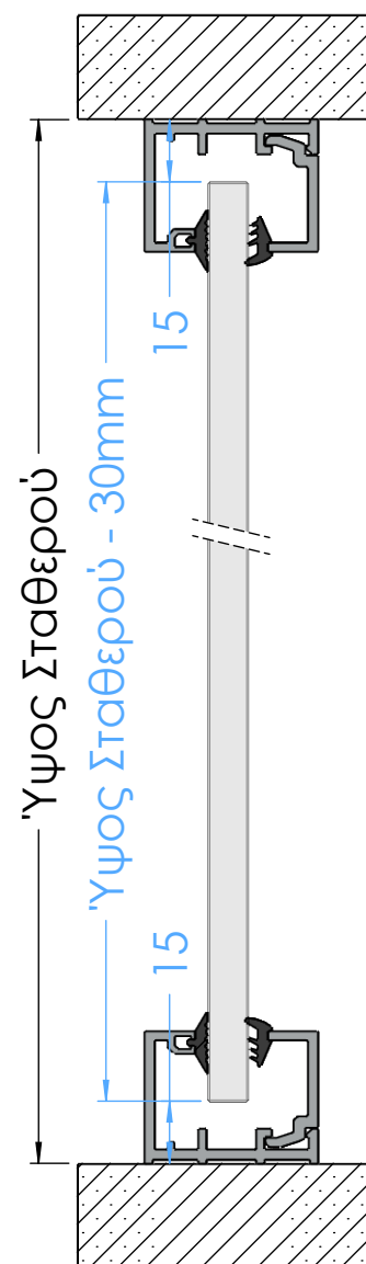
ΤΟΜΗ A-A
