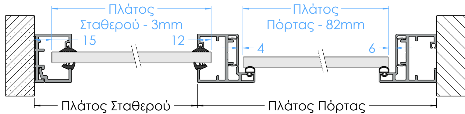
ΤΟΜΗ Κ-Κ
