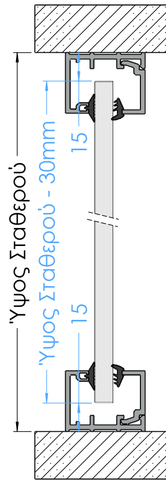
ΤΟΜΗ Α-Α
