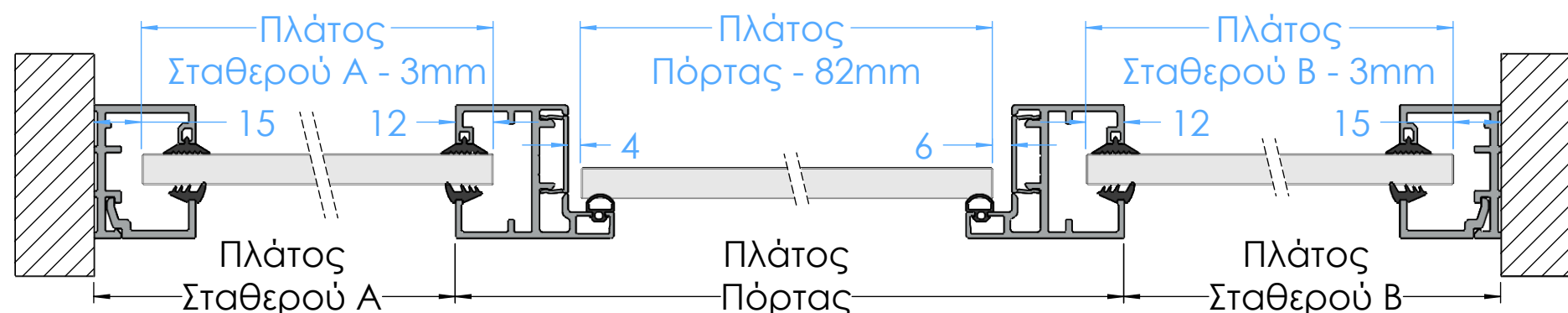
ΤΟΜΗ H-H
