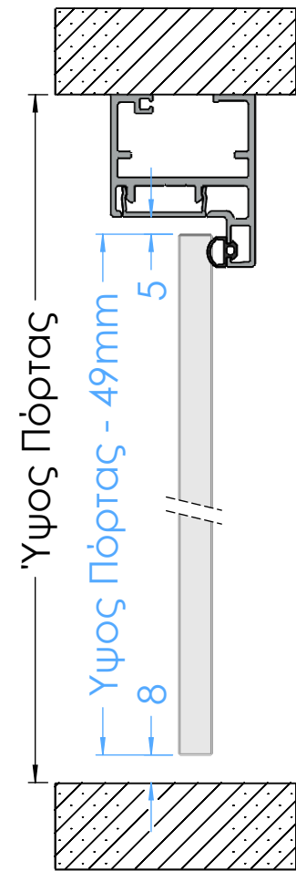
ΤΟΜΗ Β-Β
