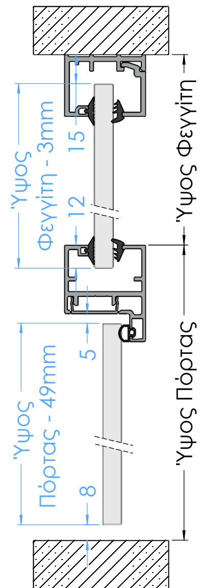
ΤΟΜΗ B-B
